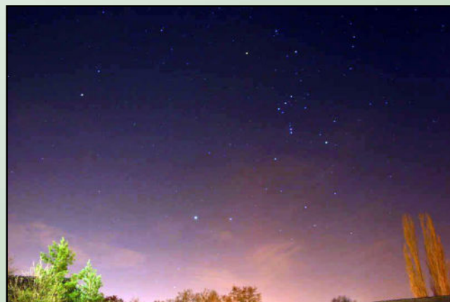
Az Orion csillagkép. Készítette Sternenhimmelhal
